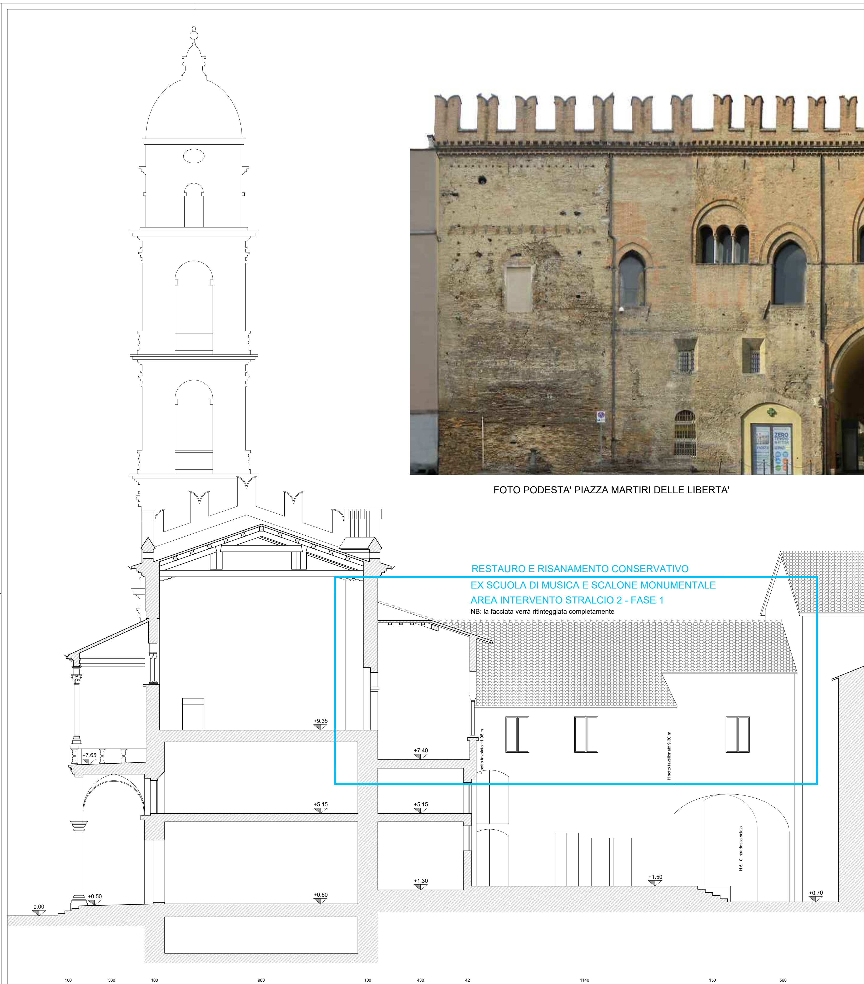
SEZIONE PODESTA' E PROSPETTO - EX ALBERGO CORONA PIAZZA MARTIRI DELLA LIBERTA'
